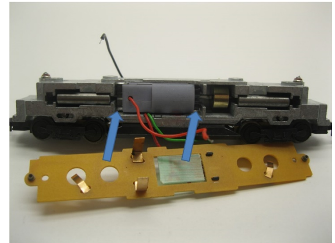
Klemmen plätzen Mount clamps Monteer de klemmen
