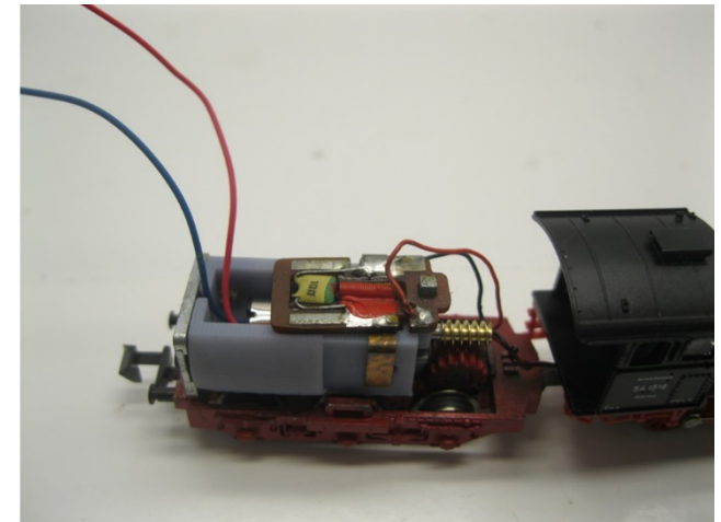
Stromanschluss platzieren Mount the power connector Plaats de contact klem
