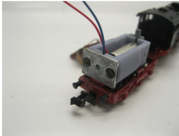
Motorhalter schrauben Screw the motor holder Schroef de motor houder
