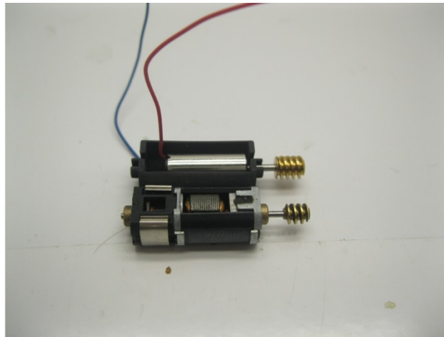
Die Metall Teile sind verklebt Metal parts are glued with Loctite or metal epoxy glue Metalen onderdelen worden gelijmd met metaallijm of epoxylijm voor metalen
