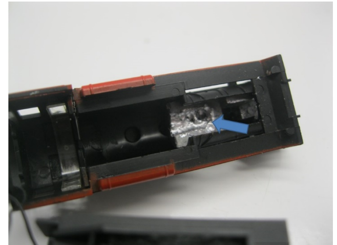
Machen Sie mit einer Fräsmaschine Platz für das Schnecken Make room for the worm wheel with a milling machine Maak wat ruimte met een frees voor het wormwiel
