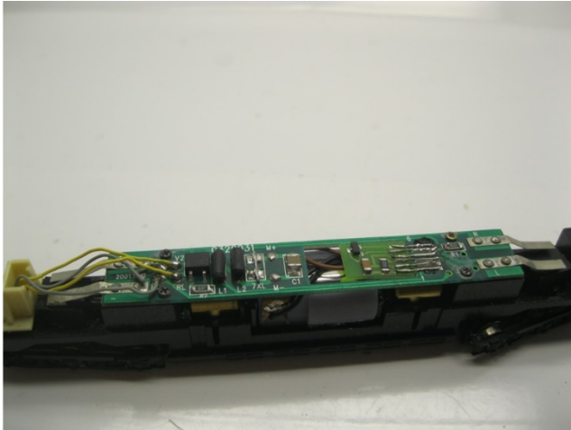
Platine plätzen und Drähte löten Place PCB and solder the wires Soldeer de draden
