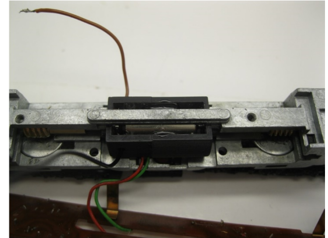
Der Motor wird mit Epoxidkleber oder Sekundenkleber in den Motorhalter eingeklebt Motorhalter eingeklebt The motor is glued into the motor holder with epoxy glue or super glue De motor wordt verlijmd in de motorhouder met secondelijm of epoxy lijm
