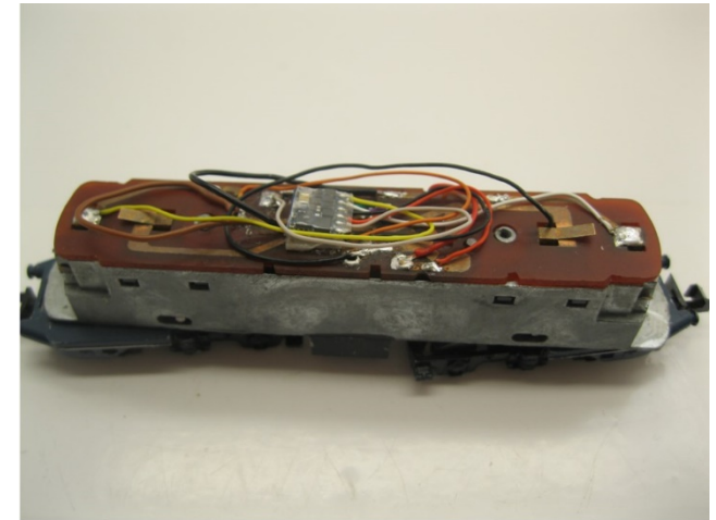
Platine platzten Place the PCB Plaats de printplaat
