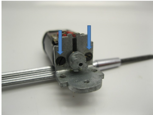
Schrauben entfernen Remove Screws Verwijder de schroeven
