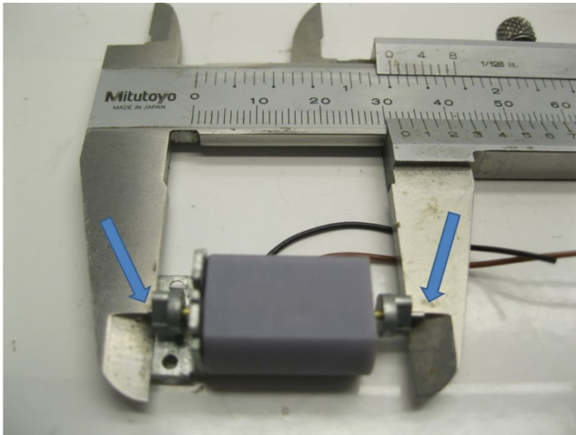
Wellen kürzen Shorten the axles Assen inkorten
