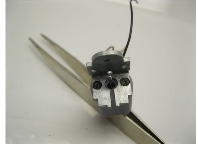
Schrauben platzieren Mount Screws Plaats de schroeven
