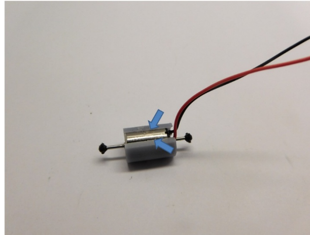
Motor in die Halterteile kleben Glue the motor in the holder parts Verlijm de motorhouder delen
