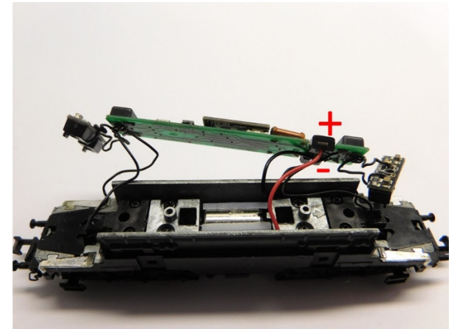
Die Drähte montieren Connect the wires Monteer de draden
