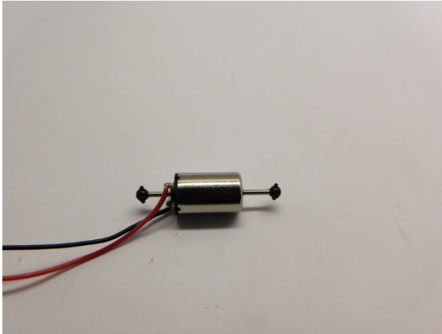
Kleben die Kardankupplungshalter Glue the cardan coupler shafts Verlijm de cardan koppelingshouders
