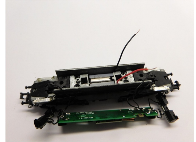
Halter platzieren Place mounts Plaats de houders
