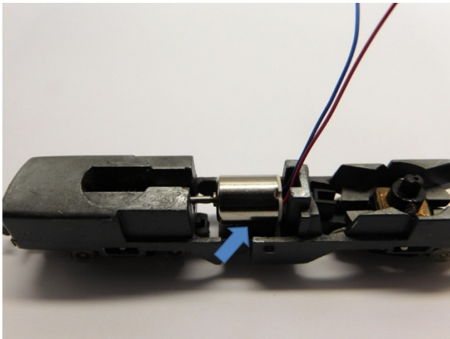
Der Motor wird mit Epoxidkleber oder Sekundenkleber in den Motorhalter geklebt The motor is glued into the motor holder with epoxy glue or super glue De motor wordt op de motorhouder verlijmd met secondelijm of epoxy lijm
