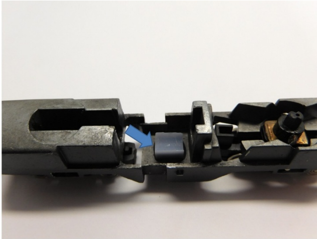
Der Motorhalter wird mit Epoxidkleber oder Sekundenkleber in den Rahmen geklebt The motor holder is glued into the frame with epoxy glue or super glue De motor houder wordt in het frame verlijmd met secondelijm of epoxy lijm
