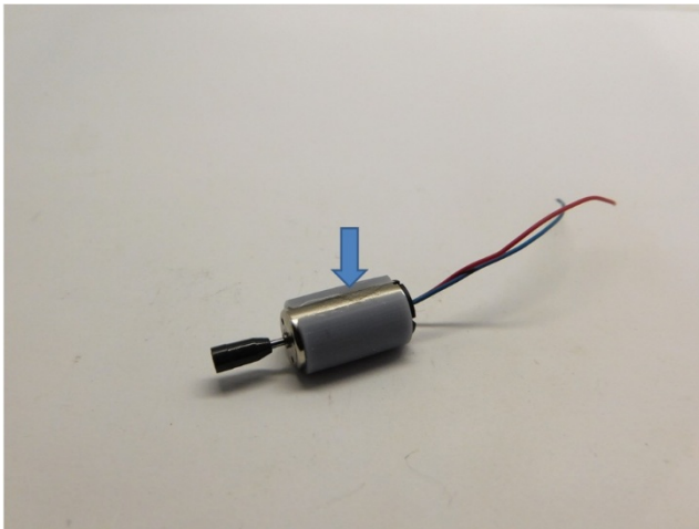
Der Motor wird mit Epoxidkleber oder Sekundenkleber in den Motorhalterteile geklebt The motor is glued into the motor holder parts with epoxy glue or super glue De motor wordt verlijmd tussen de motorhouder delen met epoxylijm of secondelijm
