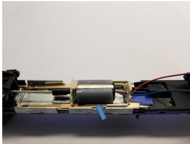
Der Motor wird geklebt The motor is glued De motor wordt verlijmd
