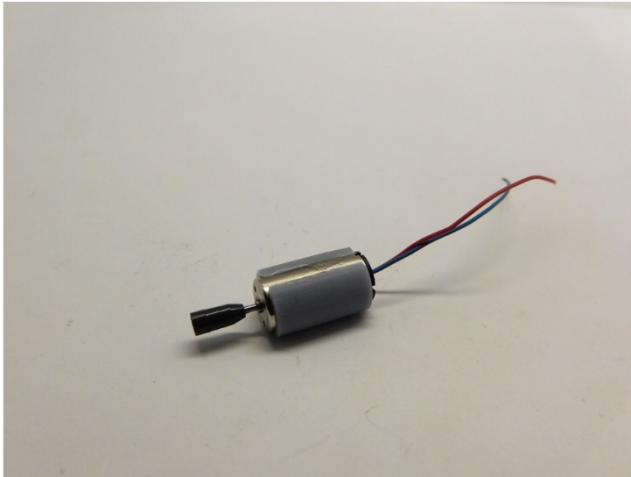
Platzieren Sie die Halter Teile und Kardankupplungshalter Mount the motor holder parts and cardan coupler shaft Plaats de motor in de motorhouder delen
