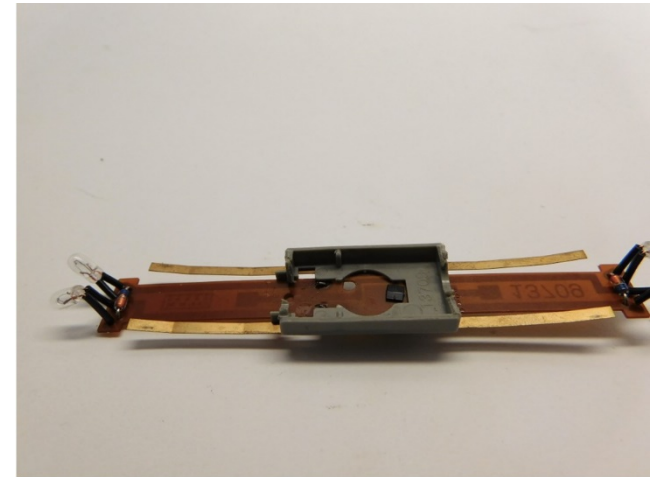
Motorhalter ändern Change motor holder Pas de motorhouder aan
