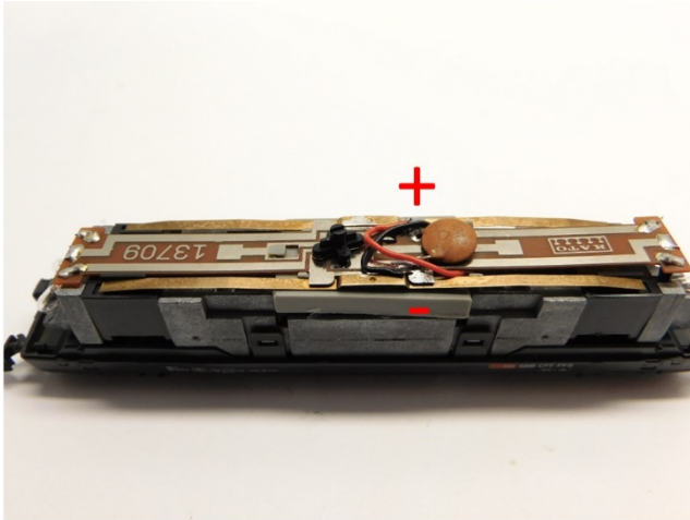
Platine platzieren & Drähte löten Mount PCB & solder the wires Soldeer de draden
