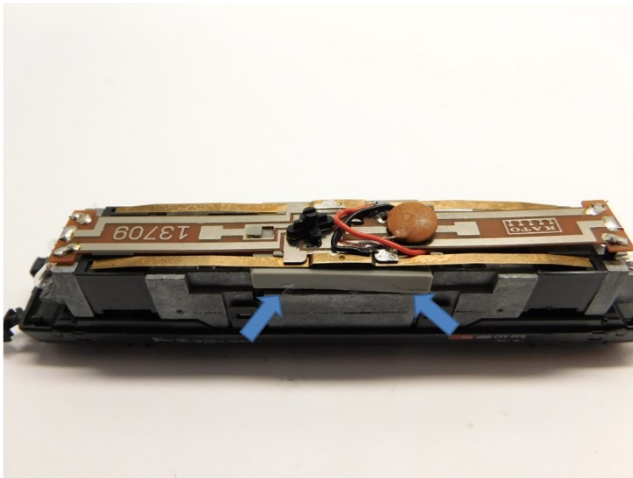
Motorhalter kleben Glue motor holder Verlijm de motor houder
