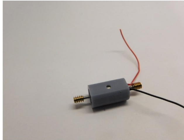
Platzieren der Motor in die Motorhalter Place the motor in the motor holder Plaats de motor in de motor houder
