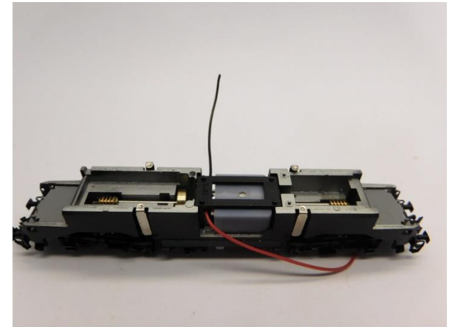
Motorklemme platzieren Mount motor clamp Plaats de motor klem
