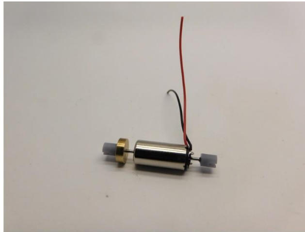
Kleben Sie die Kardankupplungen mit Sekundenkleber auf den Welle Glue the cardan couplers on the shaft with superglue Verlijm de kardankoppelingen op de as met secondelijm
