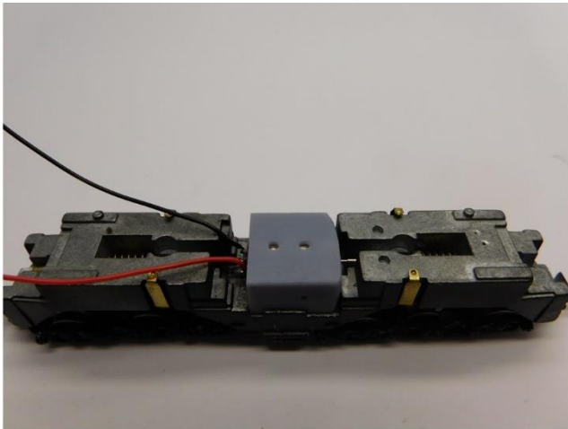
Motorhalter platzieren Mount the motor holder Plaats de motor
