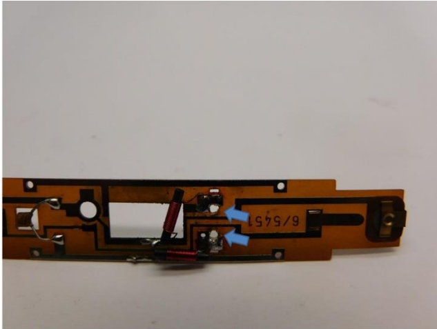
Löcher für die Drähte bohren Drill holes for the wires Boor gaten voor de draden
