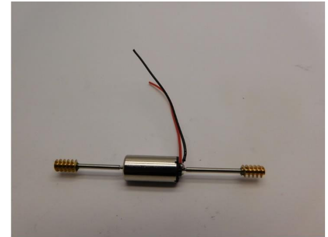
Die Drähte sind verlötet The wires are soldered De draden zijn gesoldeerd
