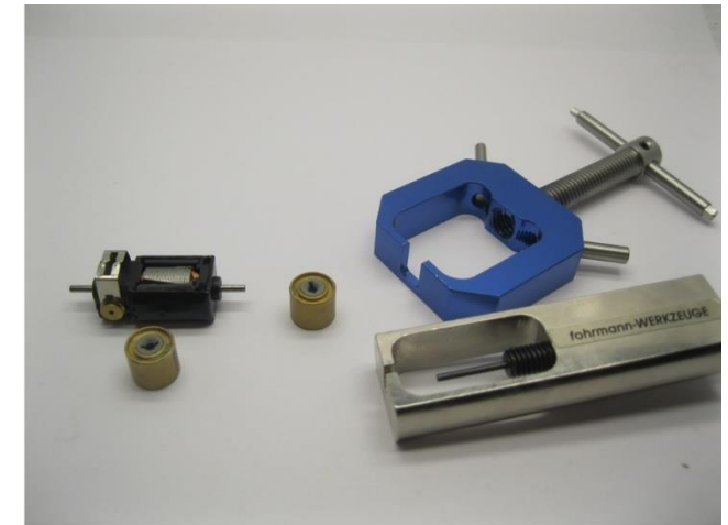
Entfernen Sie die Schwungmassen Remove the flywheels Verwijder de vliegwielen
