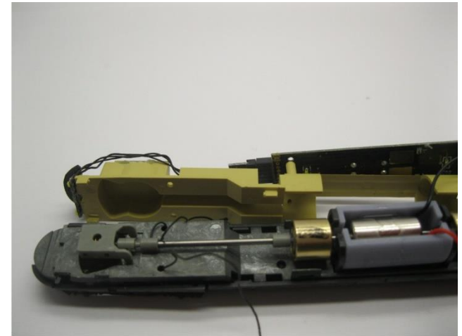
Kardanwelle platzieren Mount Cardan shaft Plaats de aandrijfjas
