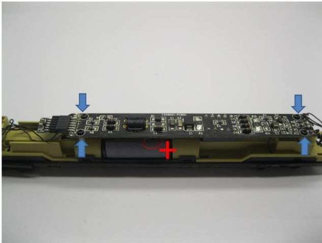
Platzieren Sie die Leiterplatte Mount the PCB Plaats de printplaat
