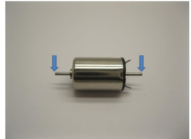
Die Achsen sind bereits gekürzt The axles are already shortened De assen zijn reeds ingekort
