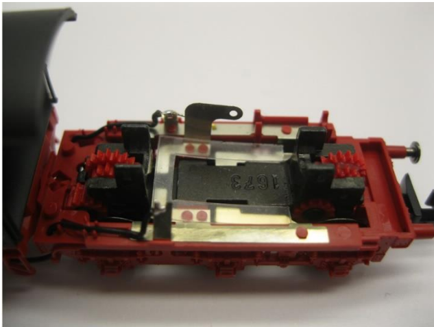
Platzieren Sie den Aufkleber zur Isolierung Mount the sticker for insulation Plaats de sticker voor isolatie
