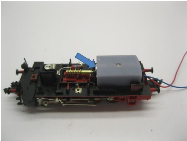
Den Motorhalter wird geklebt The motor holder is glued De motohouder wordt verlijmd
