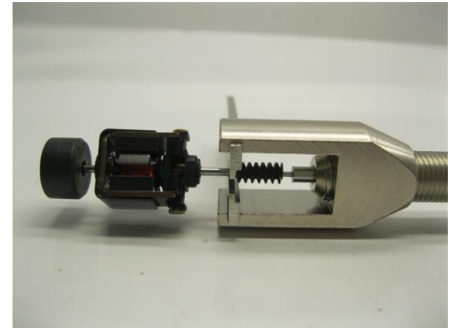
Entfernen Sie das Ritzel vom alter Motor Remove the gear from old motor Verwijder het tandwiel van de motor
