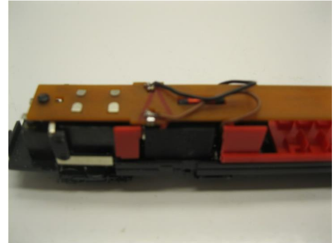
Innenraum und Platine platzieren Mount interior and PCB Plaats de inrichting en de printplaat
