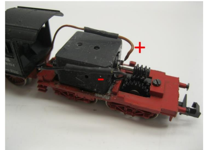
Motor platzieren und Drähte löten Mount motor and solder the wires Plaats de motor en soldeer de draden
