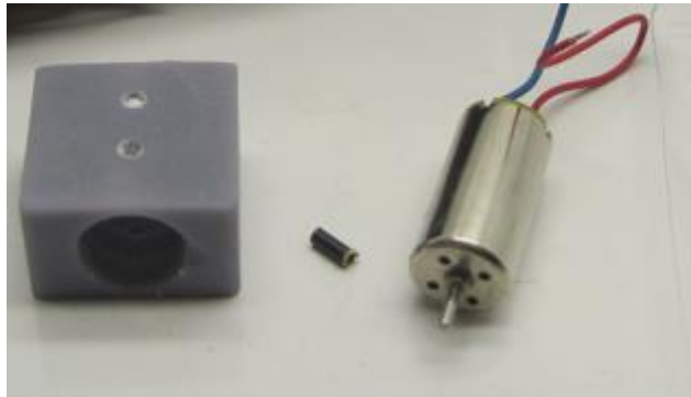
Die Teile des Bausatz Parts of the kit Onderdelen van de ombouwset
