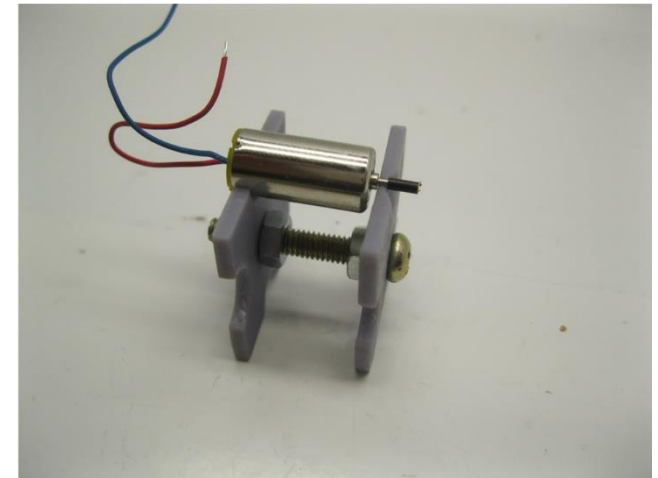
Mit einem Adapterpositionierer kann der Adapter einfach platziert werden. With an adapter positioner the adapter can be placed easily. Met een positioneer hulpstuk kan de adapter eenvoudig gemonteerd worden
