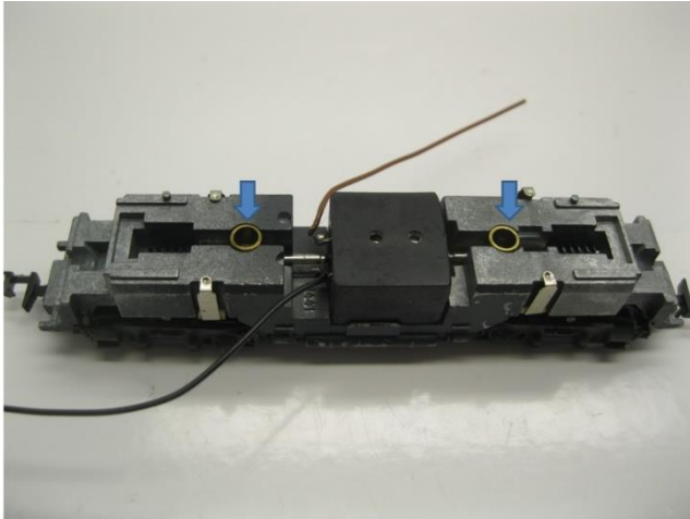
Messingbuchsen platzieren Mount brass bushings Plaats de messing lagere
