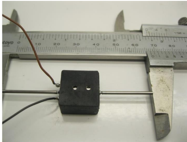
Abstand prüfen Check distance Controleer de afstand
