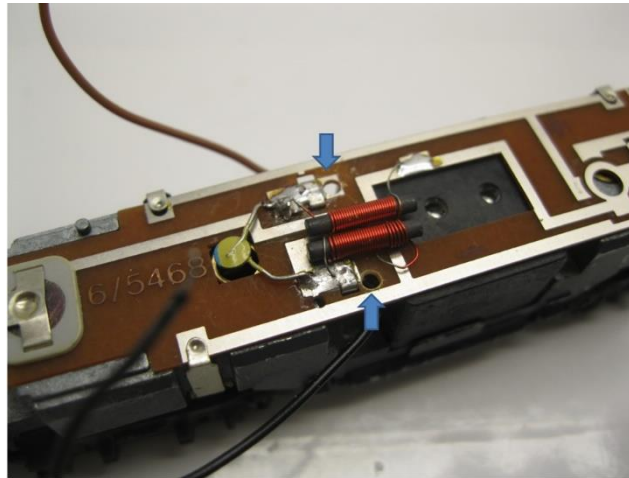
Bohren Sie 2 Löcher für die Drähte Drill 2 holes for the wires Boor 2 gaatjes voor de draden
