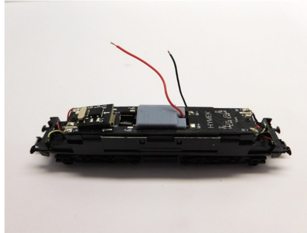
Platine platzieren Mount PCB Pkaats de printplaat
