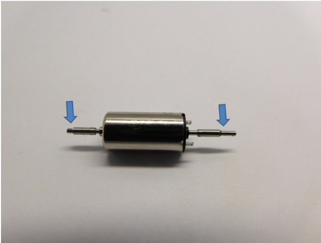
Welle kürzen mit einer Trennscheibe Shorten axles with a cutting disc Kort de assen in met een slijpschijf
