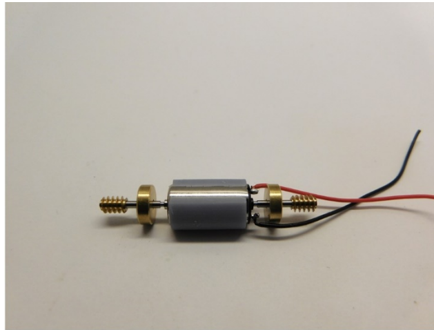
Der Motor wird mit Epoxidkleber oder Sekundenkleber zwischen den Motorhalter Teile eingeklebt The motor is glued between the motor holder parts with epoxy glue or super glue De motor wordt verlijmd in de motorhouder delen met secondelijm of epoxy lijm
