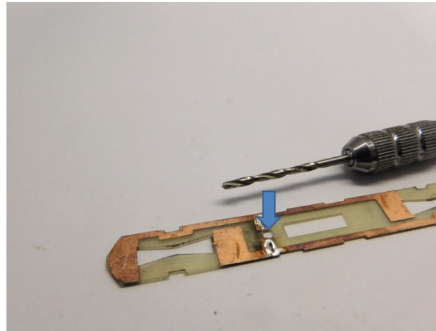
Bohren Sie ein Loch für die Drähte Drill a hole for the wires Boor een gat voor de draden
