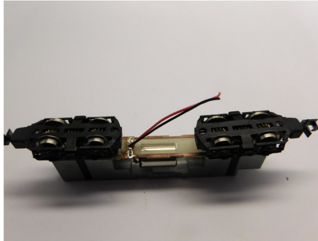
Drehgestellen platzieren Place bogies Plaats de draaistellen
