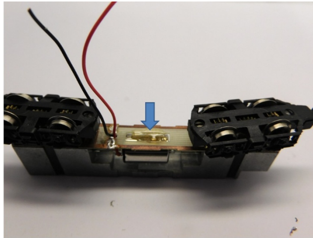
Motor kleben (Heißkleber o.ä.) Glue motor (hotmelt or other) Verlijm de motor (smeltlijm of andere)
