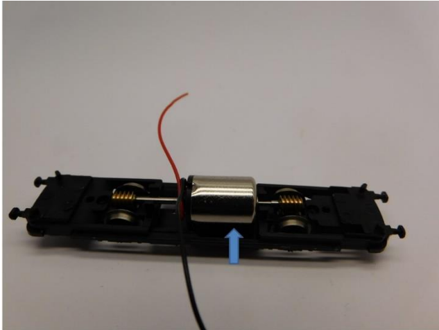
Der Motor wird mit Epoxidkleber oder Sekundenkleber in den Boden eingeklebt The motor is glued into the bottom with epoxy glue or super glue De motor wordt verlijmd op de bodem met secondelijm of epoxy lijm
