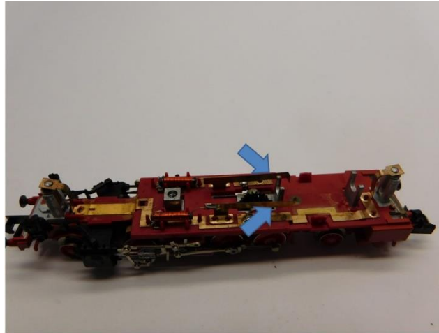
Die Kontakte müssen gekürzt werden The contacts must be shortened De contacten moeten ingekort worden
