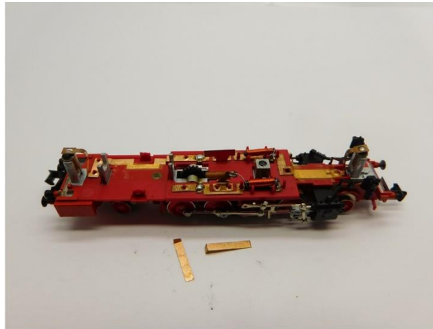
Die Kontakte müssen gekürzt werden The contacts must be shortened De contacten moeten ingekort worden
