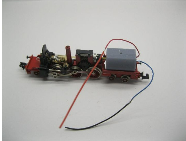
Löten Sie die Drähte. Da sie zu kurz sind, werden sie zuerst verlängert Solder the wires. Because they are too short, they are extended first Soldeer de draden. Omdat ze te kort zijn worden ze eerst verlengd
