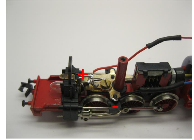
Löten Sie die Drähte. Da sie zu kurz sind, werden sie zuerst verlängert Solder the wires. Because they are too short, they are extended first Soldeer de draden. Omdat ze te kort zijn worden ze eerst verlengd
