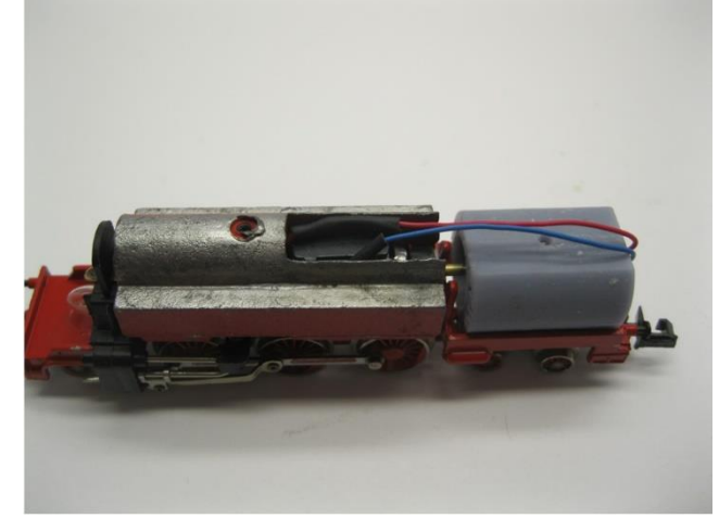
Gewicht platzieren Mount the weight Plaats het gewicht
