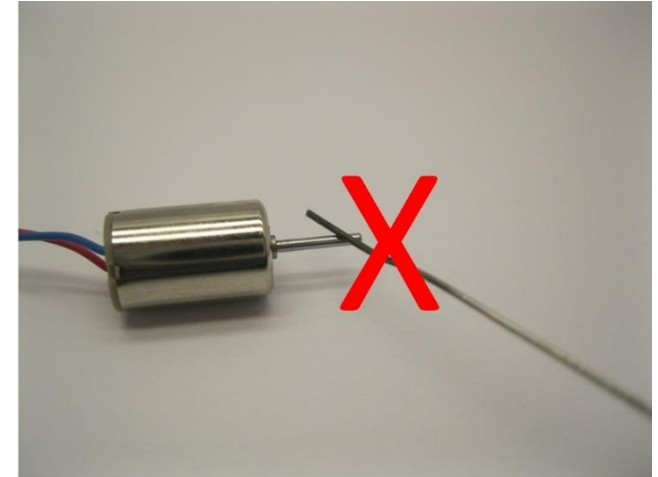
Tragen Sie Klebstoff auf die Innenseite des Teile auf. Tragen Sie keinen Kleber auf die Achse auf Apply glue on the inside of the part. Don't apply glue on the axle Plaats alleen lijm aan de binnenzijde van de onderdelen. Plaats geen lijm op de as
