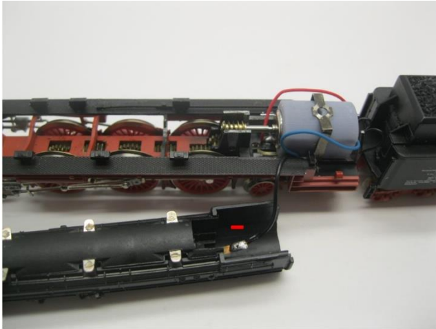
Löten Sie die Dräht Solder the wire Soldeer de draad
