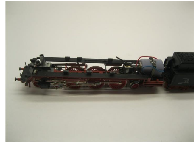
Umlaufblech platzieren Mount the footplate Plaats de voetplaat
