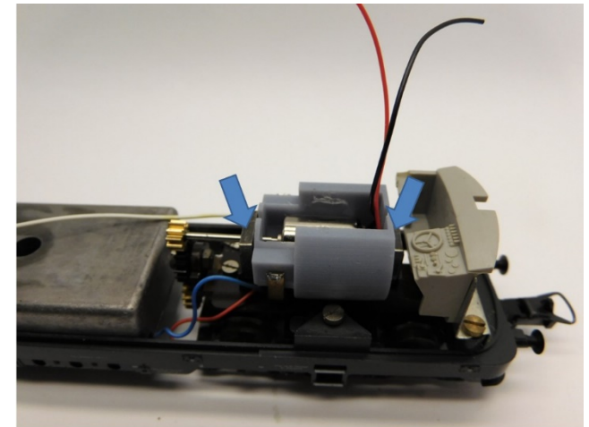
Klemme platzieren Mount clamps Plaats de klemmen
