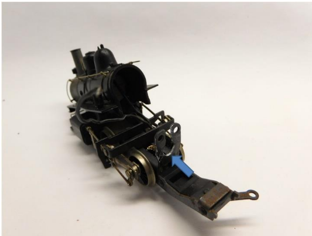
Loch vergrößern Enlarge the hole Vergroot het gat
