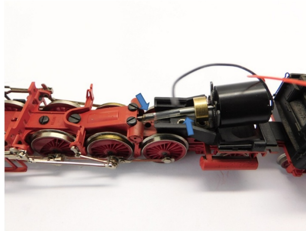
Der kupplung wird mit Sekundenkleber geklebt The coupler is glued with super glue De koppeling is verlijmd met secondelijm
