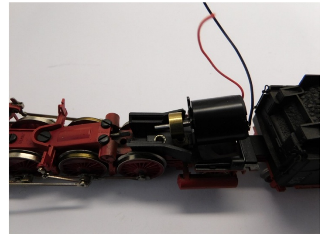
Passgenauigkeit prüfen Test fit Probeer of het past
