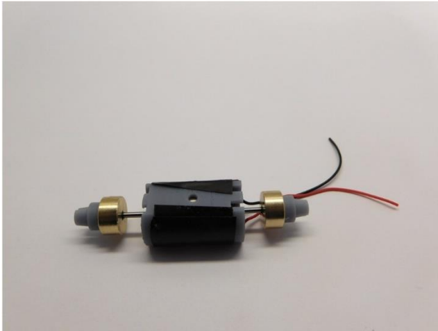
Isolierband vom alten Motor platzieren Mount insulating tape from old motor Plaats de isolatietape van de oude motor
