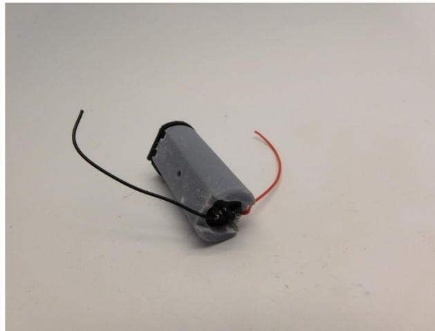
Platzieren Sie den Motor in die Motorhalter Mount the motor in the motor holder Plaats de motor in de motor houder
