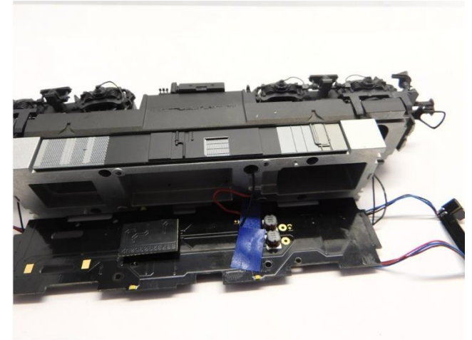
Kontakten isolieren Isolate the contacts Isolleur de contacten
