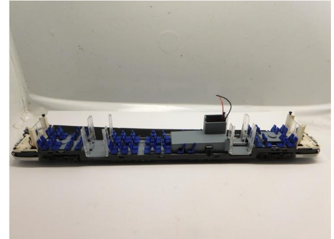
Innenrichtung platzieren Place the interior Plaats de inrichting
