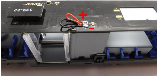
Drähte löten Solder the wires Soldeer de draden
