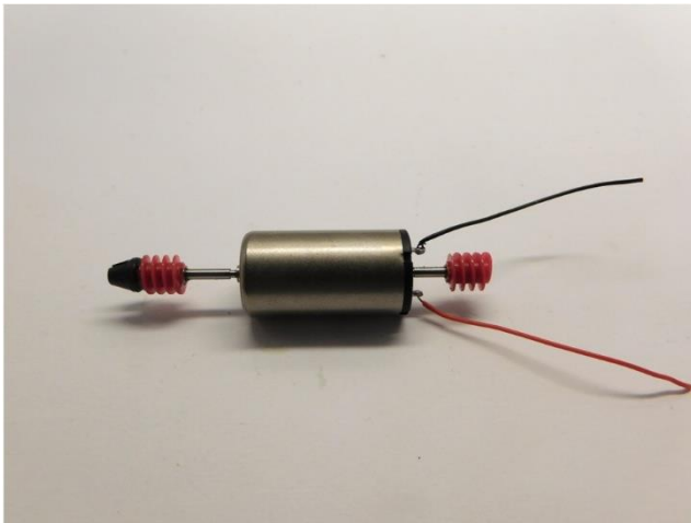
Kleben Sie die Schnecken Glue the worm gears Verlijm de wormwielen
