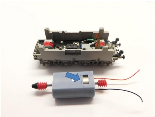
Dieses Teil von der Motorhalterung entfernen Remove this piece from the motor holder Verwijder dit stukje uit de motorhouder
