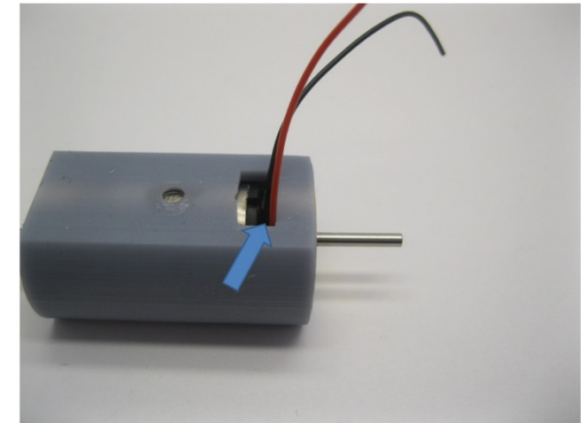
Legen Sie Spannung an den Motor und prüfen Sie, dass kein Kurzschluss zwischen den Kontakten und dem Schwungmasse vorliegt Apply voltage to the motor and check that there is no short circuit between the contacts and the flywheel Sluit de spanning aan en controleer of er geen kortsluiting tussen de contacten en het vliegwiel plaats vindt
