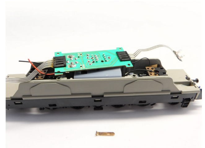
Alter Motorkontakte entfernen Remove old motor contacts Verwijder de oude motorcontacten
