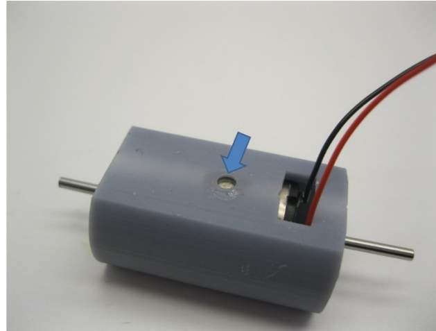
Der Motor wird mit Epoxidkleber oder Sekundenkleber in den Motorhalter eingeklebt The motor is glued into the motor holder with epoxy glue or super glue De motor wordt in de motorhouder verlijmd in de motorhouder met secondelijm of epoxy lijm
