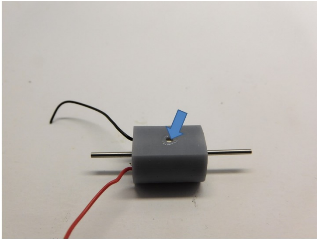
Der Motor wird mit Epoxidkleber oder Sekundenkleber in den Motorhalter eingeklebt The motor is glued into the motor holder with epoxy glue or super Glue De motor wordt in de motorhouderverlijmd met secondelijm of epoxy lijm
