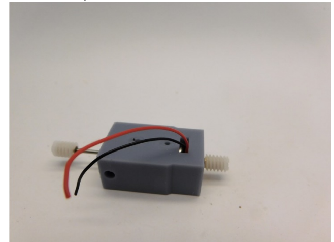
Platzieren Sie die Schnecken Mount the worm gears Monteer de wormwielen
