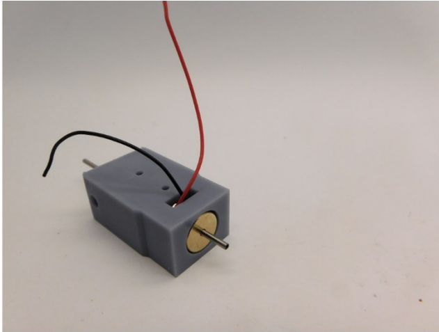
Platzieren Sie die zweite Schwungmasse Mount the second flywheel Plaats het tweede vliegwiel
