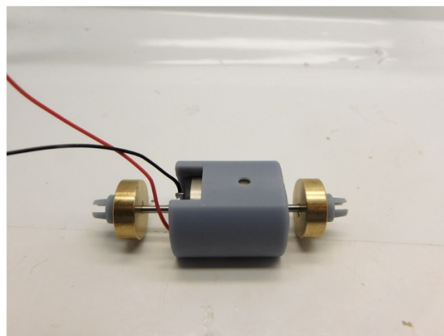
Platzieren Sie die Kardankupplungen Mount the cardan couplers Plaats de kardan koppelingen
