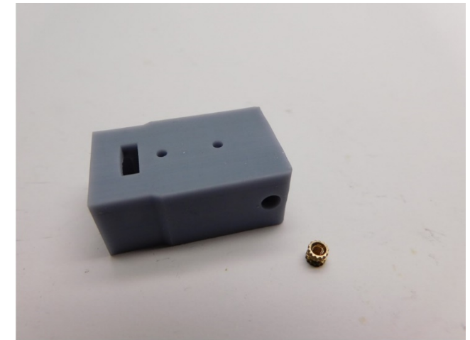
Die Messinginsert wird mit Sekundenkleber in den Motorhalter eingeklebt The brass insert is glued into the motor holder with superglue De messing insert wordt met secondelijm verlijmd in de motor houder
