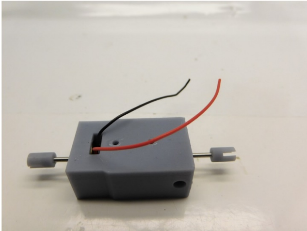
Platzieren Sie die Kardan Kupplungen Mount the cardan couplers Monteer de kardan koppelingen
