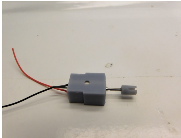
Platzieren Sie die Kardankupplung Mount the cardan coupler Monteer de cardan koppeling
