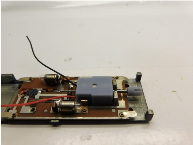
Platzieren Sie den Motor auf die Platine Mount the motor on the PCB Monteer de motor op de printplaat
