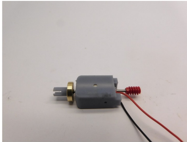
Platzieren Sie die Schnecke & Kardan Kupplung Mount the worm gear and cardan coupler Monteer het wormwiel en de kardan koppeling
