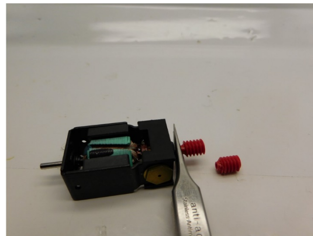
Sie brauchen diese Teile wieder. Diese werden mit einer Pinzette entfernt You need the parts again. They can be removed with tweezers Je hebt deze onderdelen wederom nodig. Het kan met een pincet verwijderd worden
