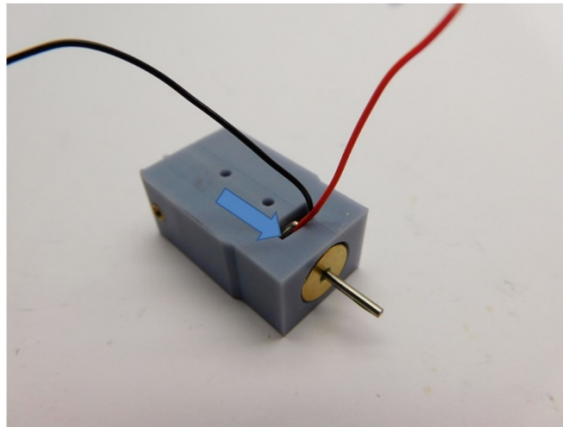
Legen Sie Spannung an den Motor und prüfen Sie, dass kein Kurzschluss zwischen den Kontakten und dem Schwungmasse vorliegt Apply voltage to the motor and check that there is no short circuit between the contacts and the flywheel Sluit de spanning aan en controleer of er geen kortsluiting is tussen de contacten en het vliegwiel
