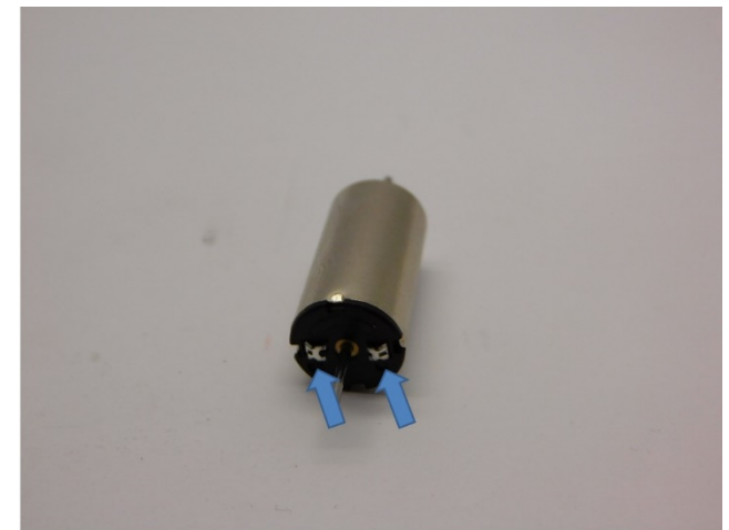
Biegen und kürzen Sie die Lötlippen! Bend and shorten the soldering lips! Buig en kort de soldeerlippen in!
