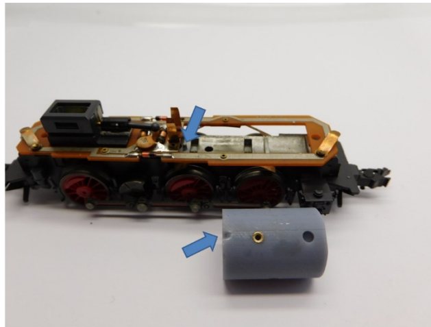
In der Motorhalterung muss eine Nut angebracht werden A slot must be made in the motor holder Brenge een kleine sleuf aan in de houder
