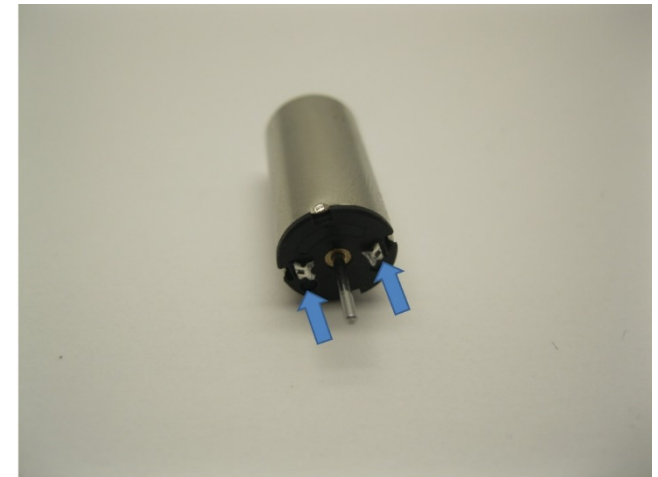
Biegen und kürzen Sie die Lötlippen! Bend and shorten the soldering lips! Buig de soldeerlippen en kort ze in!
