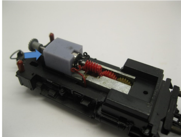
Der Motor wird mit Sekundenkleber geklebt The motor is glued with super Glue De motor wordt met secondelijm verlijmd
