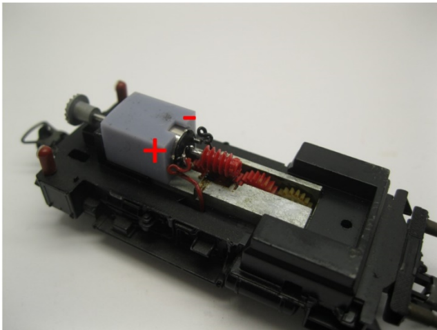
Motor platzieren und löten Sie die Drähte Mount the motor and solder the wires Plaats de motor en soldeer de draden
